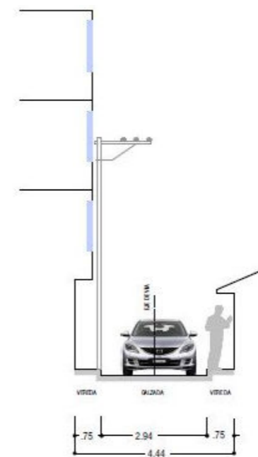
SECCIÓN A-A
